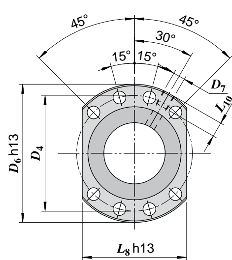
Flange type 2 ( d_0 > 40 mm)
